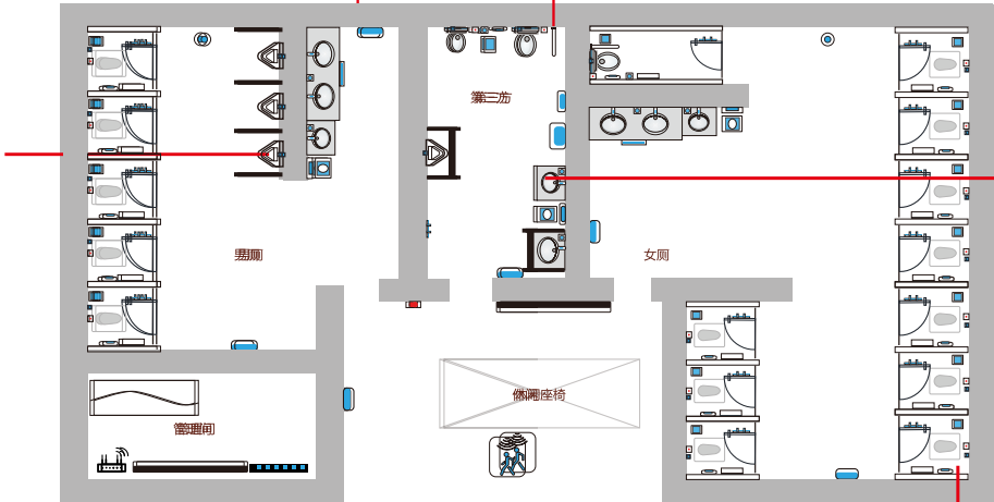
瑞沃智慧公厕示意图
